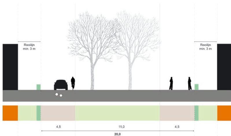
Profiel 2: woonhof
