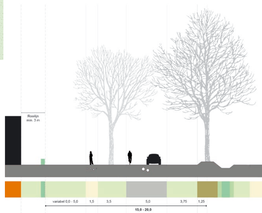
Profiel 1: hoofdontsluiting
