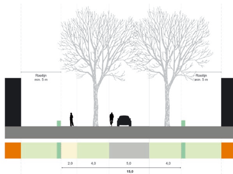
Profiel 1: Hoofdontsluiting
