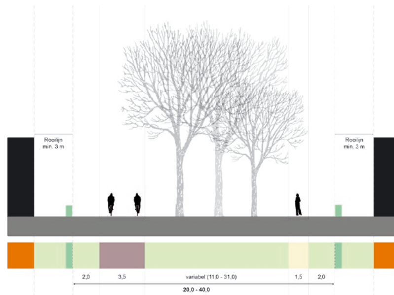
Profiel 3: Fietspad
