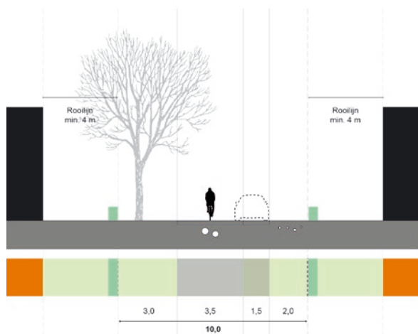
Profiel 2: Woonstraat
