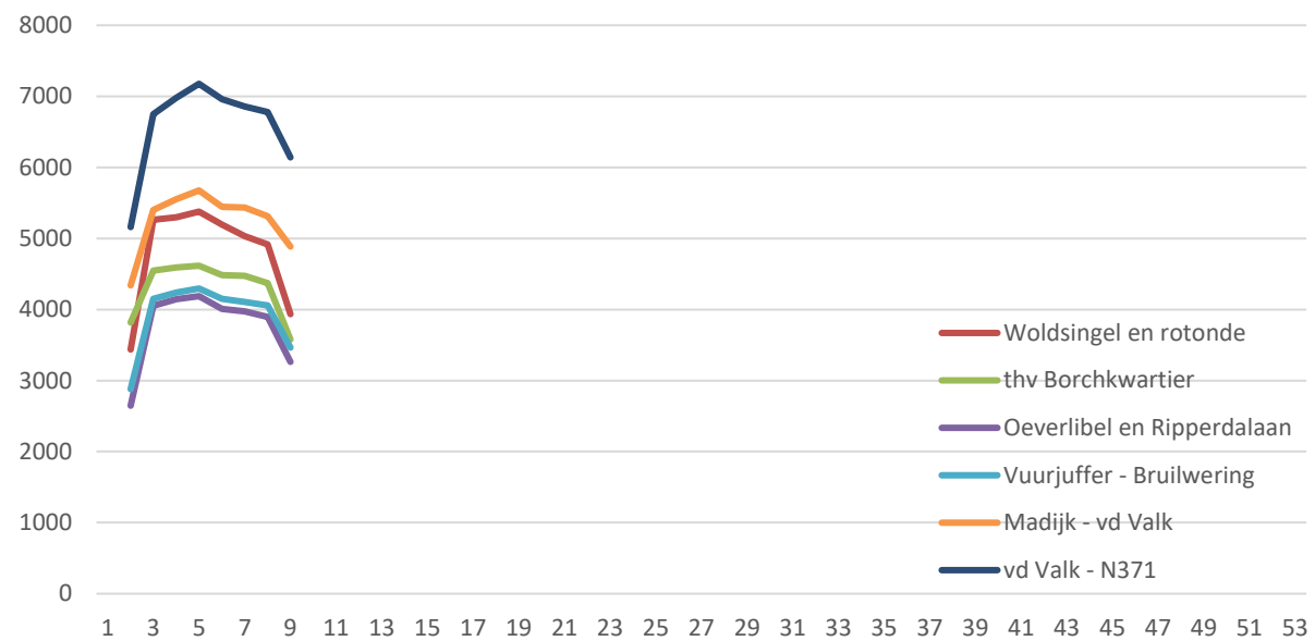
2025 24 uur werkdaggemiddelde
