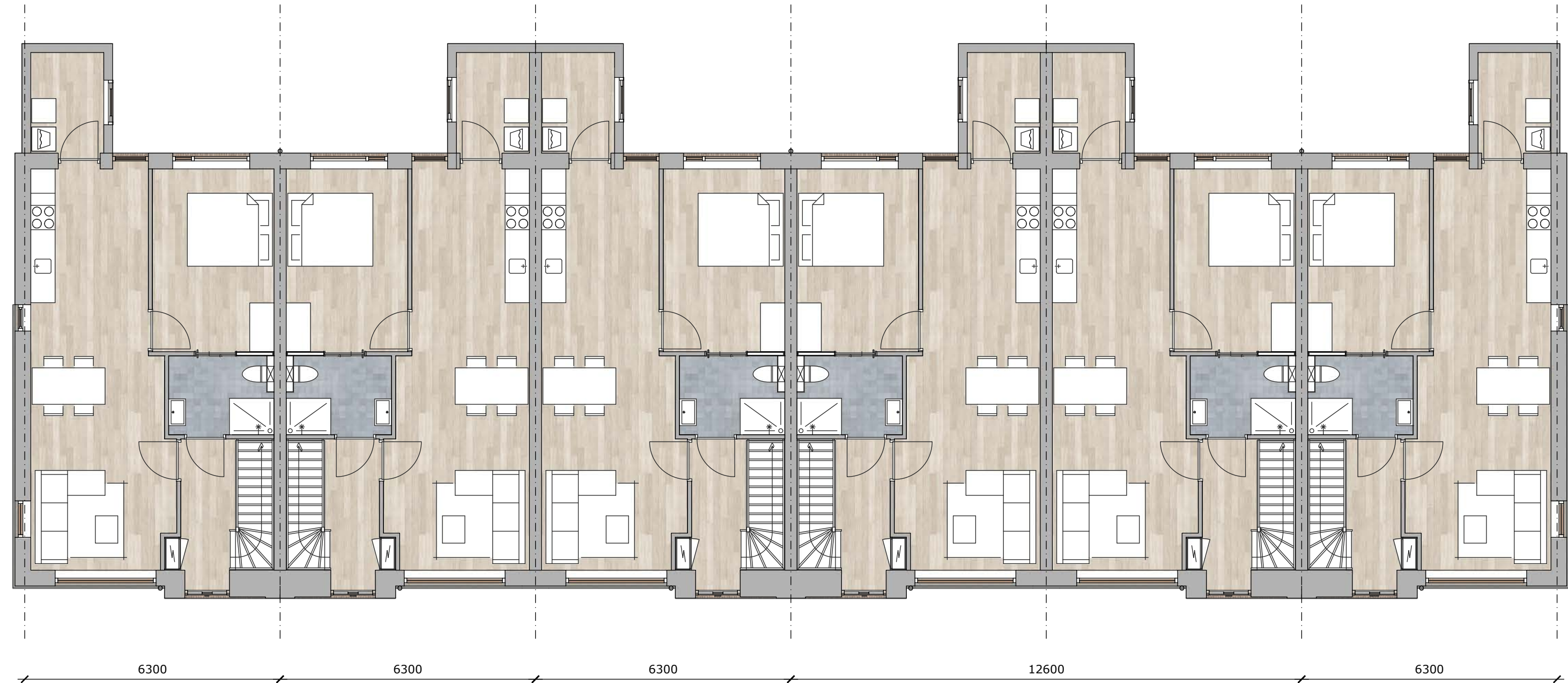
begane grond schaal 1:100
