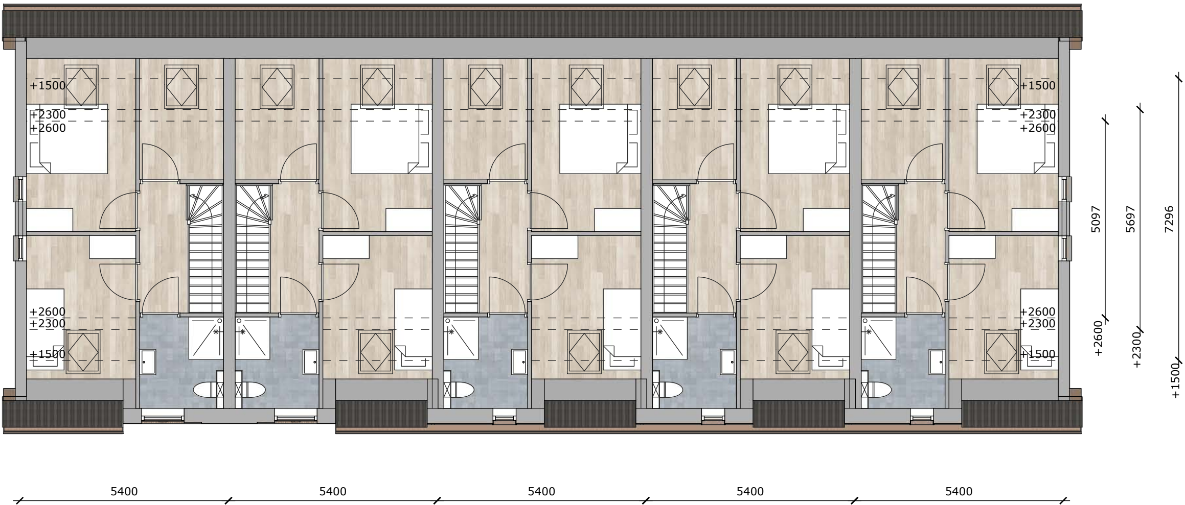
verdieping schaal 1:100
