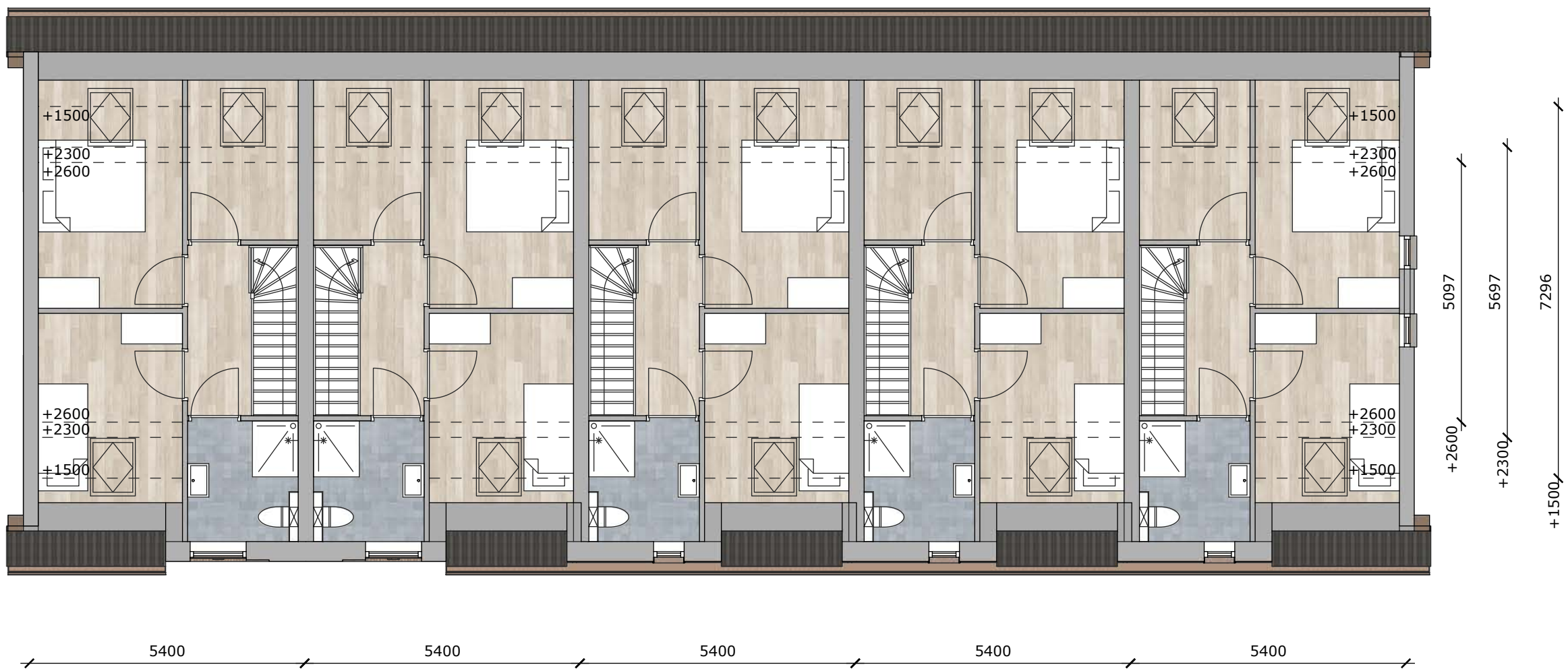
verdieping schaal 1:100
