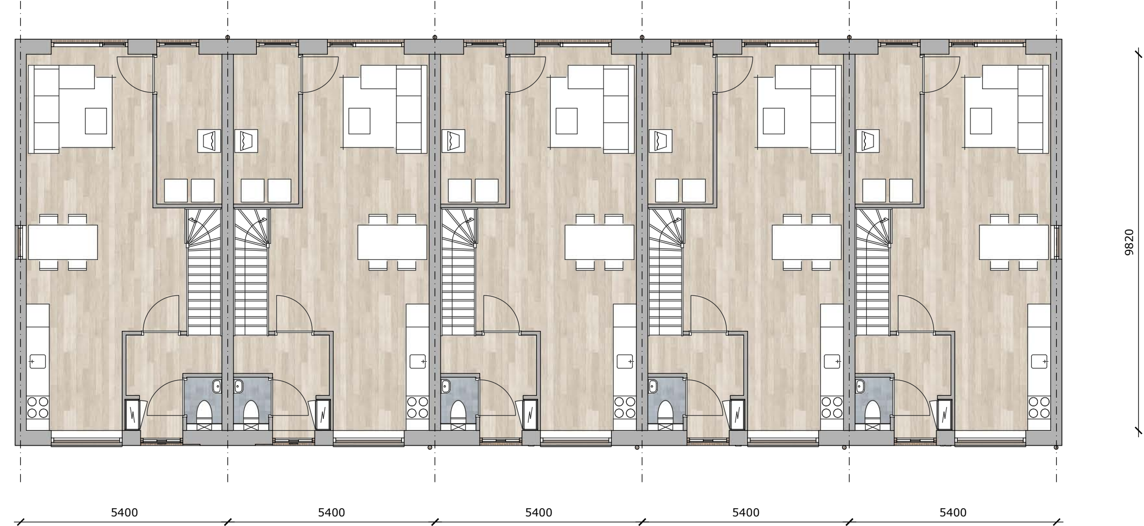
begane grond schaal 1:100
