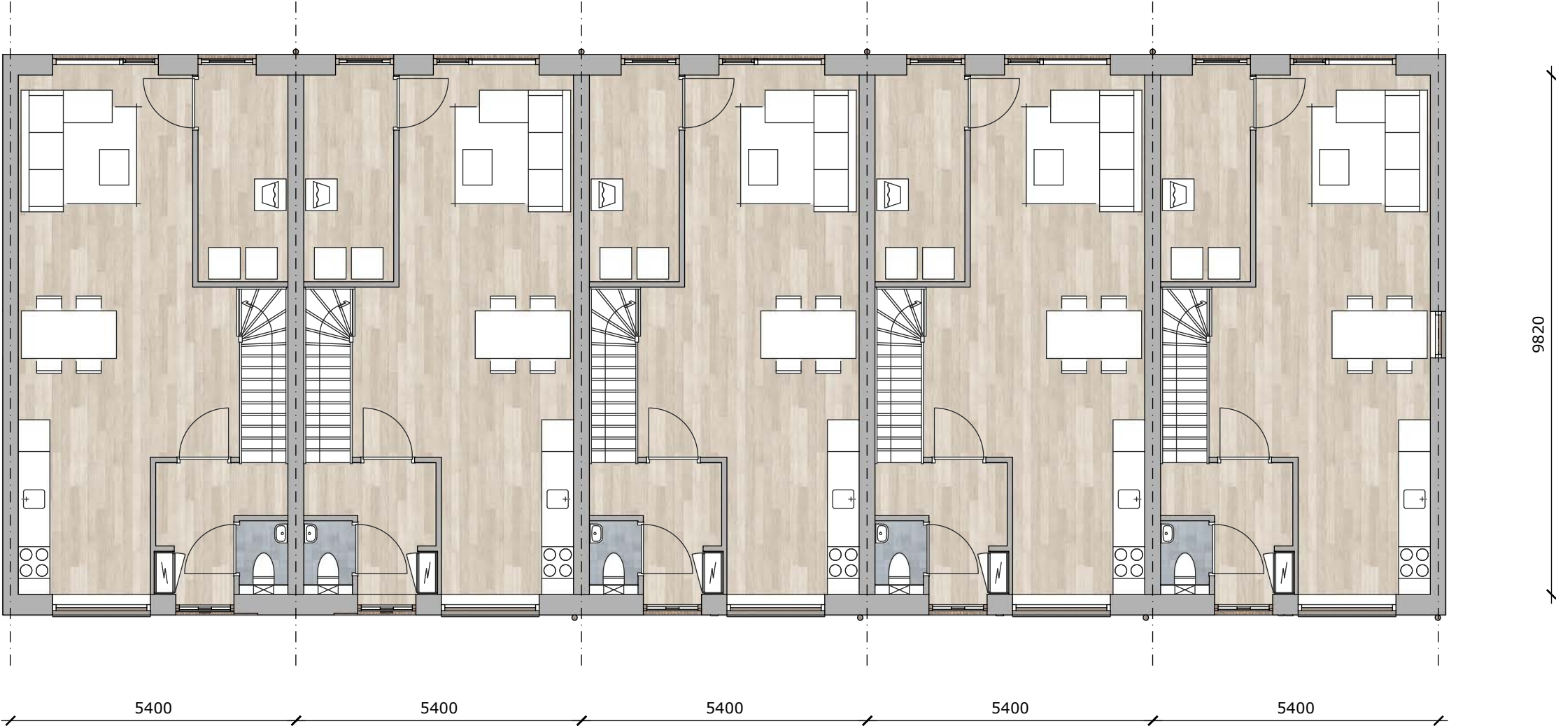
begane grond schaal 1:100
