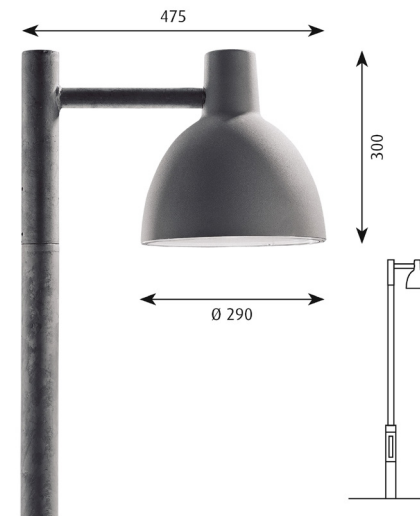
Verlichting; mast uitgevoerd in gegalvaniseerd staal of gelijkwaardig, afgestemd op transferium
