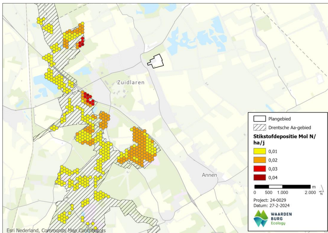
Figuur 4.3 Spreiding van projectbijdrage ter plaatse van Natura 2000-gebied Drentsche Aa (Bron: AERIUS-calculator, versie 2023.1).
