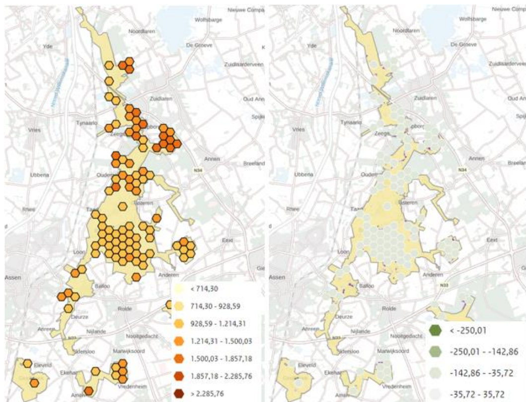
Figuur 4.1 Huidige achtergronddepositie Drentsche Aa (links) en de ontwikkeling van de achtergronddepositie sinds 2020 (Bron AERIUS-Monitor, 2024).
