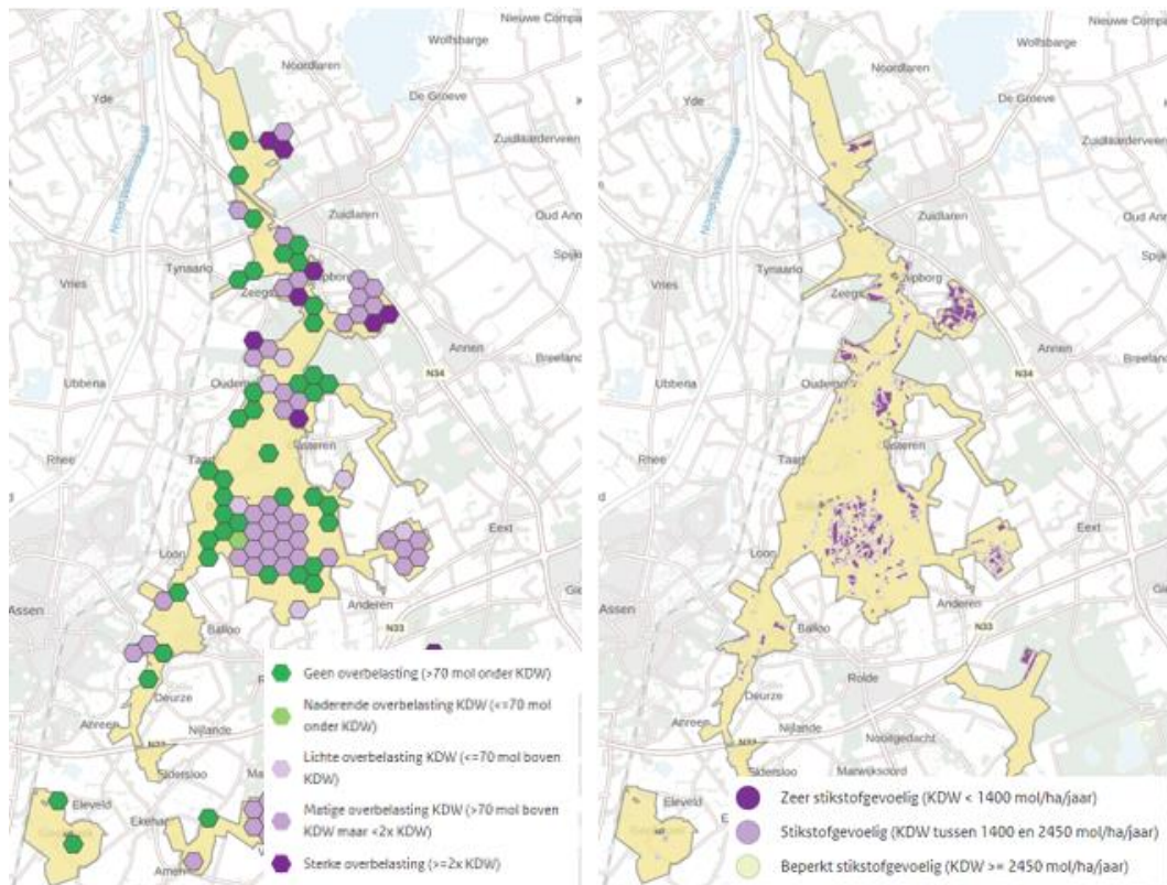
Figuur 4.2 Afstand tot de KDW in Drentsche Aa (mate van overschrijding, links) en ligging voor stikstof gevoelig habitat (rechts) (Bron AERIUS-monitor, 2024).
